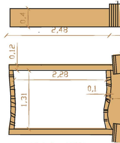
مخطط توضيحي لحوض البئر.
