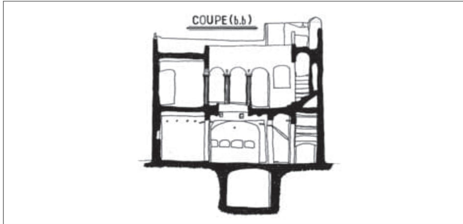
مقطع B-B
