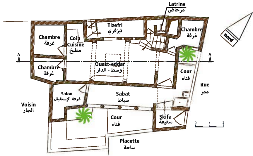
مخطط الطابق الأرضي PLAN R.D.C.
