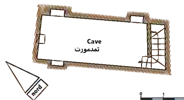
مخطط الطابق السفلي PLAN SOUS-SOL
