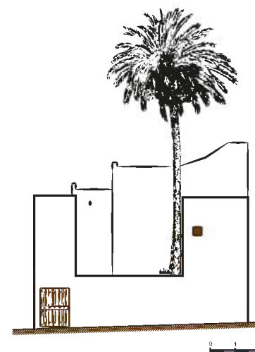
Façade الواجهة الشرقية
