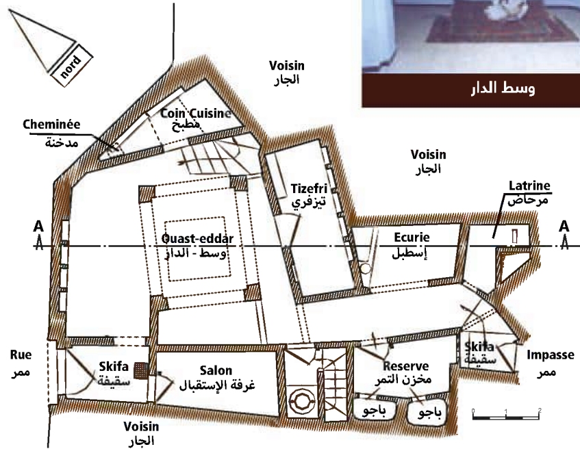
مخطط الطابق الأرضي PLAN R.D.C.
