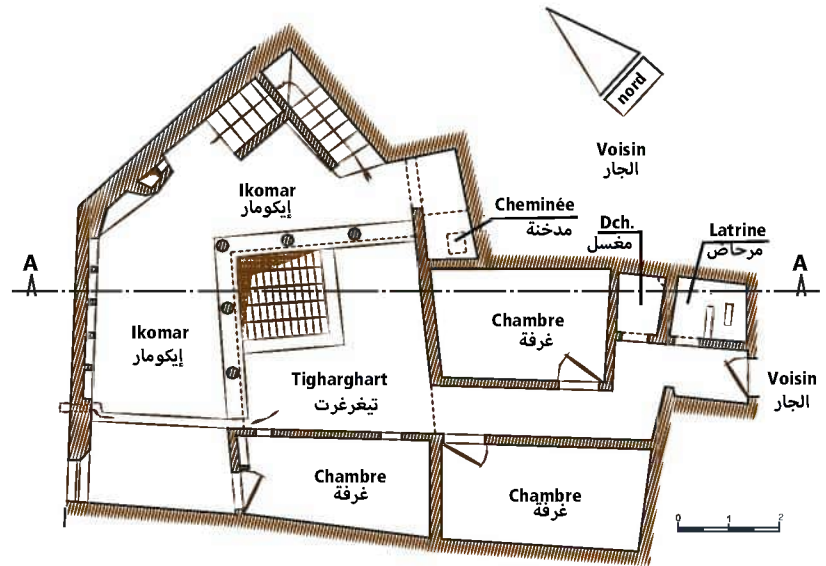
مخطط الطابق الأول PLAN ETAGE
