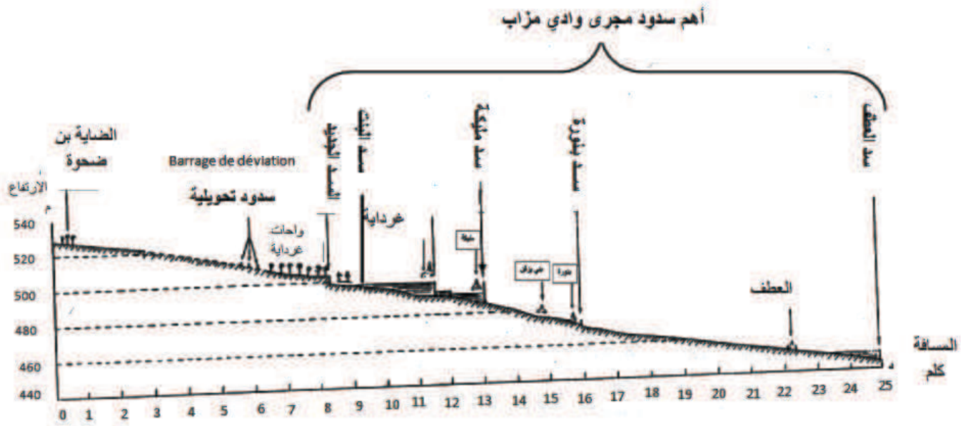
الشكل رقم (2): انخفاض مستوى وادي مزاب من الشمال الغربي إلى الجنوب الشرقي وموقع أهم السدود منه
